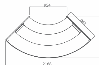
Angolo 90° solo con vetri dritti versione tavola fredda
