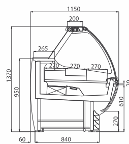
VETRINA PRALINERIA VENTILATA
