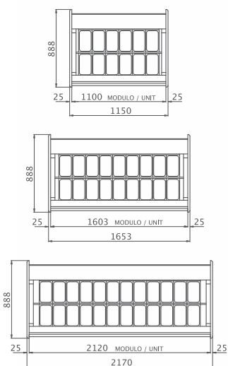
Lunghezze moduli per tutte le versioni
